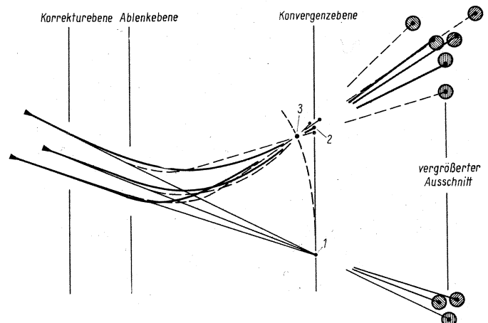
Bild 1. Konvergenzkorrektur vor der Ablenkebene
