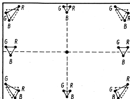
Bild 4. Konvergenzfehler bei der 110°-Röhre
