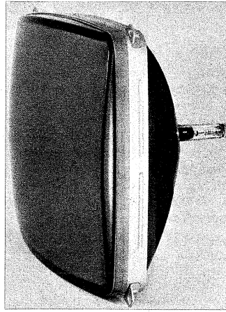
Bild 2. a = Kurz, flach und gedrun-gen ist die 110°-Schwarzweißbild-röhre A 61-120 W. b = Relativ lang und etwas unproportioniert wirkt die MW 36-24 mit dem damals schräg eingesetzten Elektroden-system und Ionenfalle
