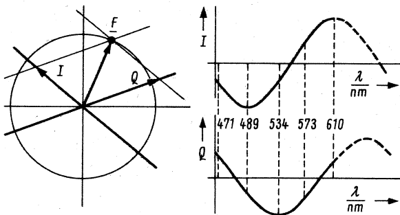
Farbdifferenzsignale Farbfernsehen
