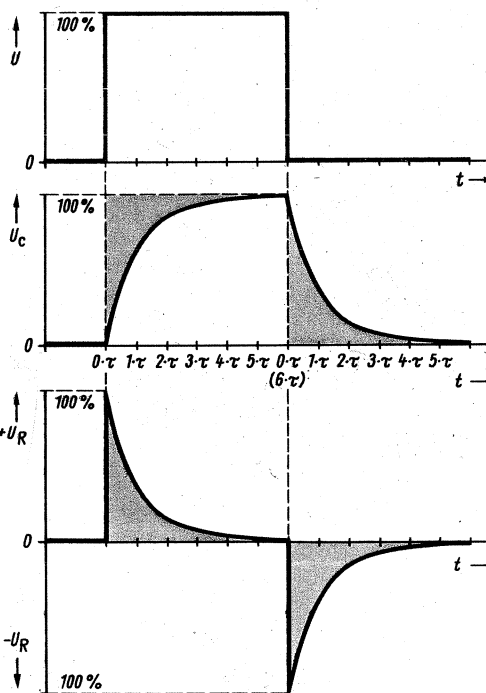
Bild 3.9. Spannungsteilung am RC-Glied
