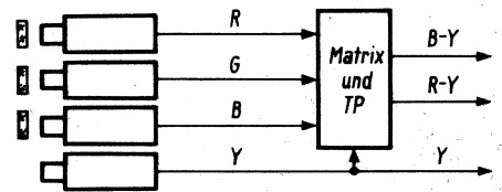
Vierröhren-Farbkamera Analogie: Auge mit vier Rezeptoren (1 Modulator mit 3 Dominatoren)
