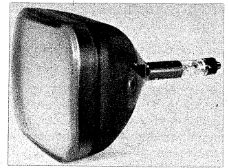
Bild 2. a = Kurz, flach und gedrun-gen ist die 110°-Schwarzweißbild-röhre A 61-120 W. b = Relativ lang und etwas unproportioniert wirkt die MW 36-24 mit dem damals schräg eingesetzten Elektroden-system und Ionenfalle
