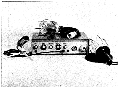
Steuergerät und Stroboskoplampen für psychedelisches Licht der Heimann GmbH, Wiesbaden-Dotzheim
