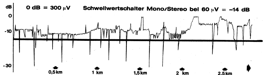
Bild 4. Feldstärke-Diagramm, aufgenommen bei einer Fahrt
