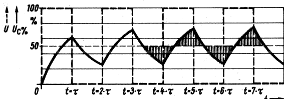
Bild 3.8. Verformung einer Rechteckimpulsfolge durch ein RC-Glied; Kondensatorspannung in Abhängigkeit von der Zeit
