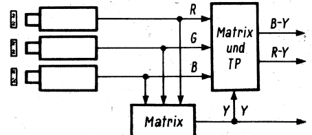
Dreiröhren-Farbkamera Analogie: Auge mit drei Rezeptoren
